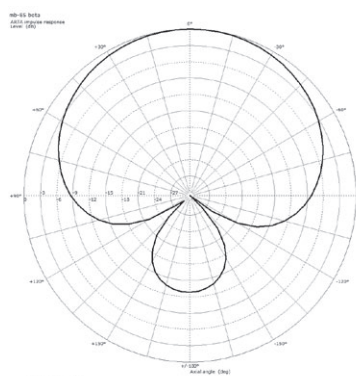
Polardiagramm @ 1 kHz
