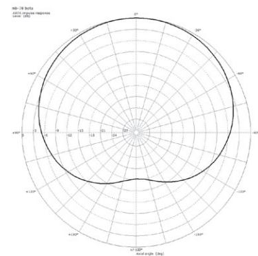
Polardiagramm @ 1 kHz
